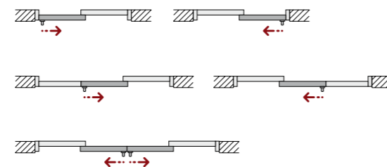
Zobrazení způsobů otvírání zdvižně posuvných dveří:
